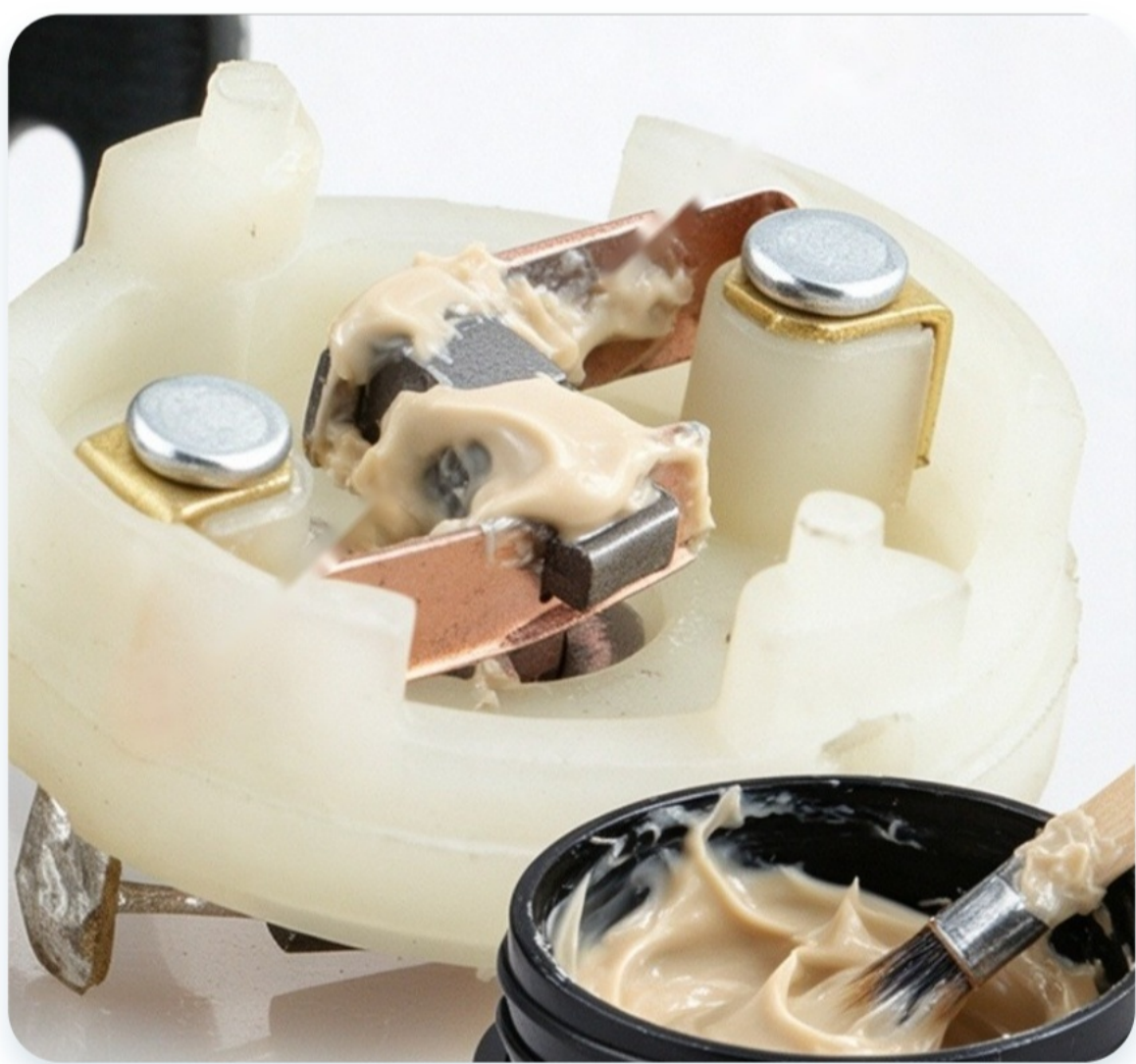
电刷-换向器摩擦副施脂示意
